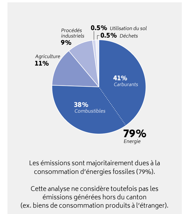
Répartition actuelle des émissions de GES par habitant (données 2015)
