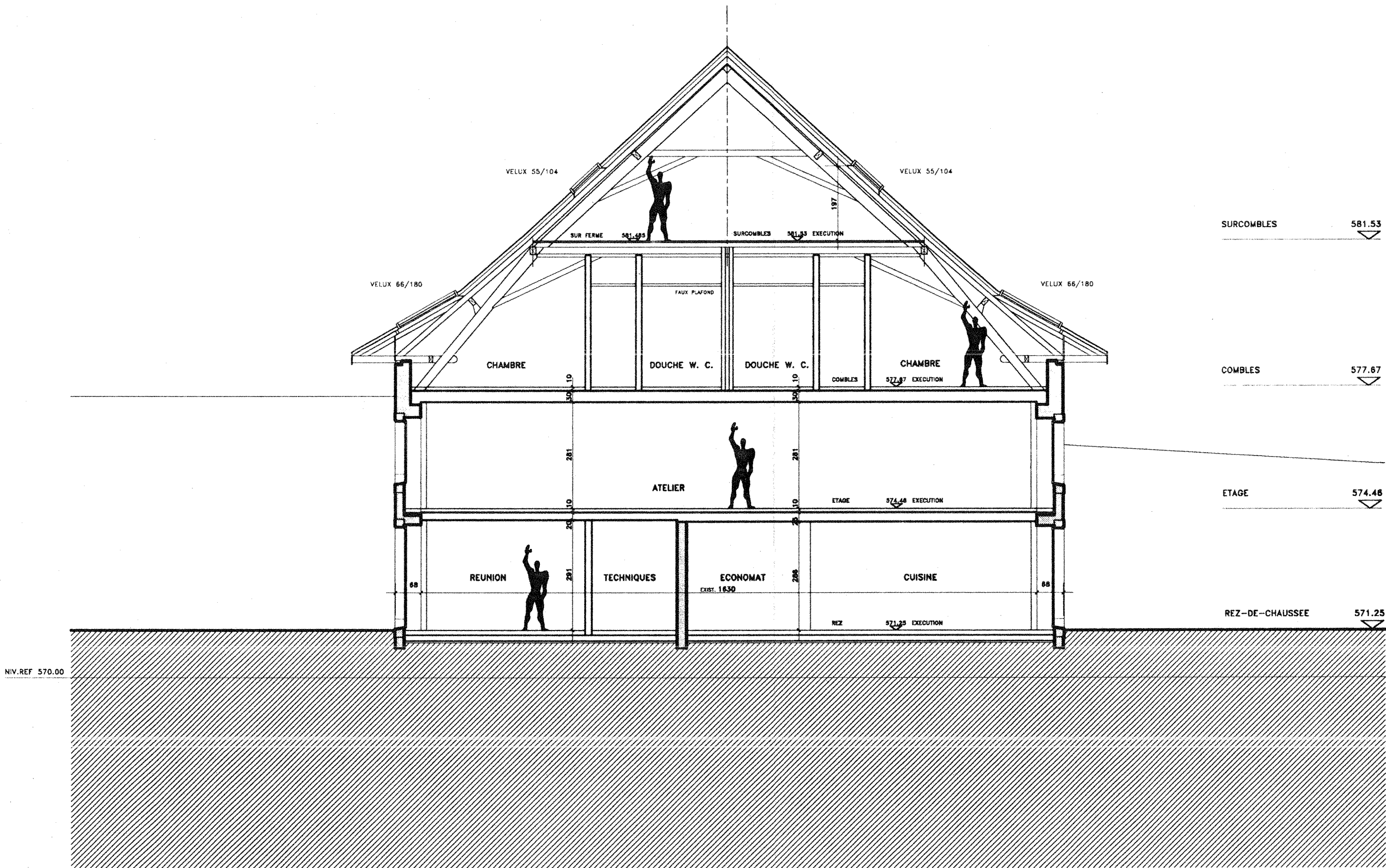
COUPE C-C
