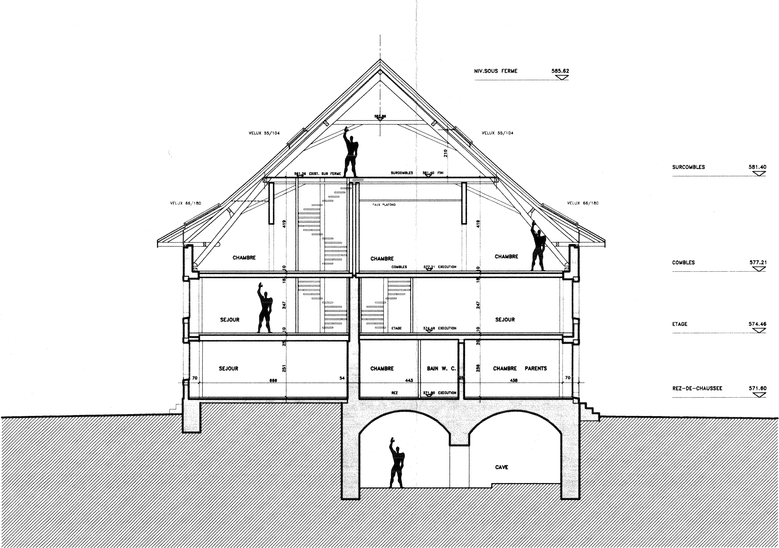
COUPE A-A
