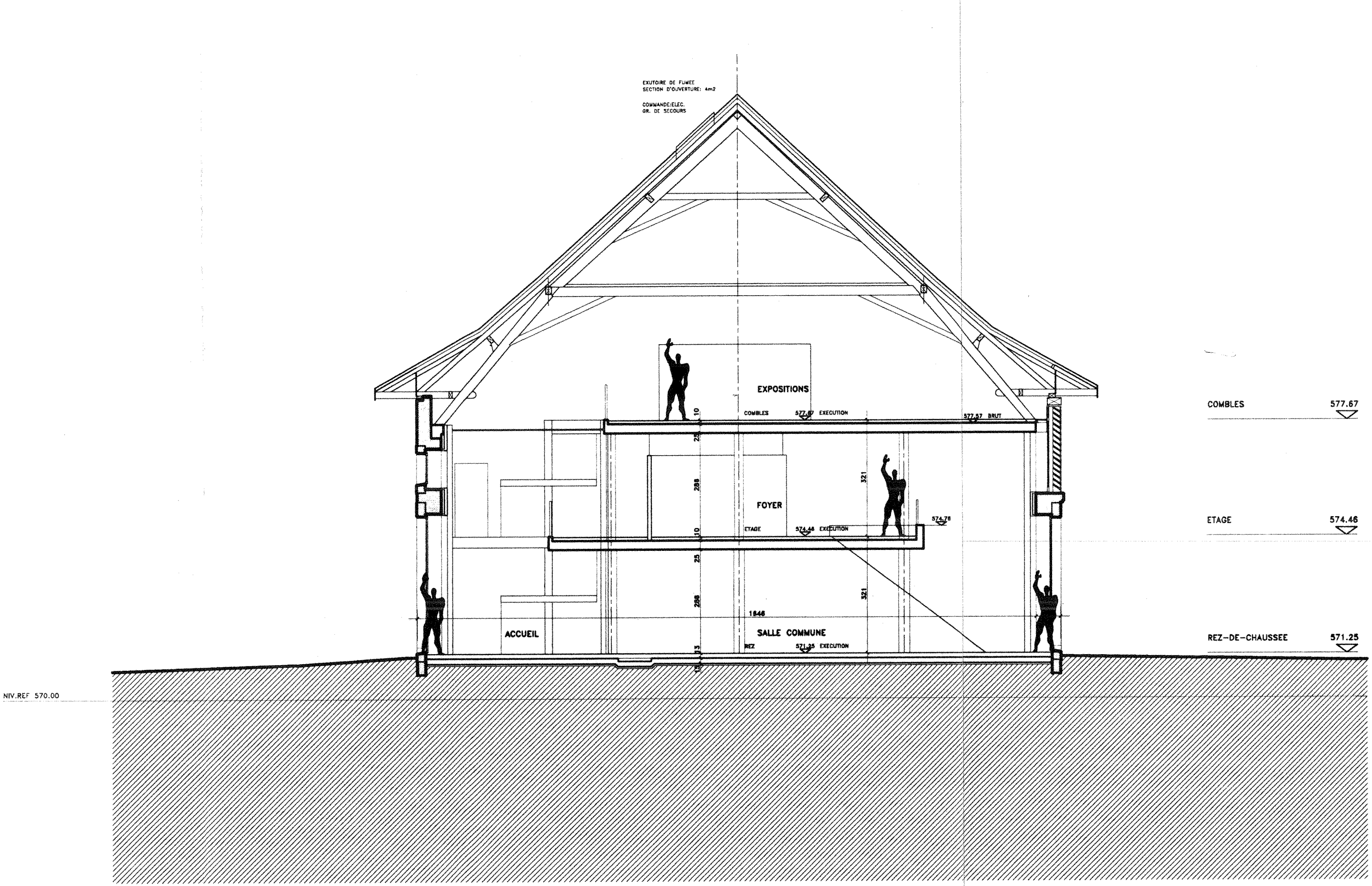
COUPE B-B
