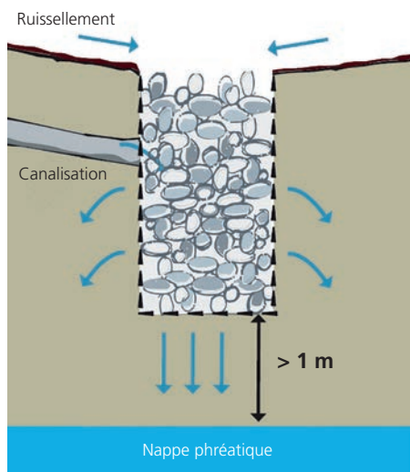
Schéma d'un fossé d'infiltration
