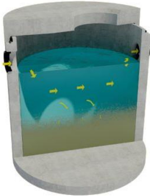
Séparateur à hydrocarbures + filtre à coalescence
