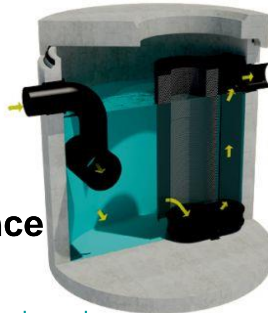
Séparateur à hydrocarbures
