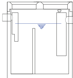
Figure 8: déshuileur avec décanteur incorporé.
