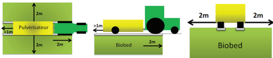
Figure 12: dimensionnement minimal.
