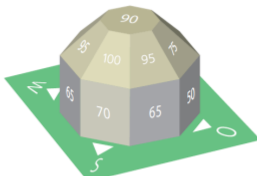
graphique indiquant le rendement annuel en fonction de l'orientation
