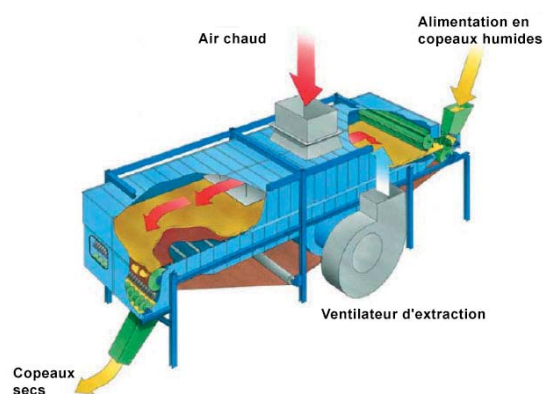
Principe du séchoir à bande (W. Kunz dryTec AG. 2005).
