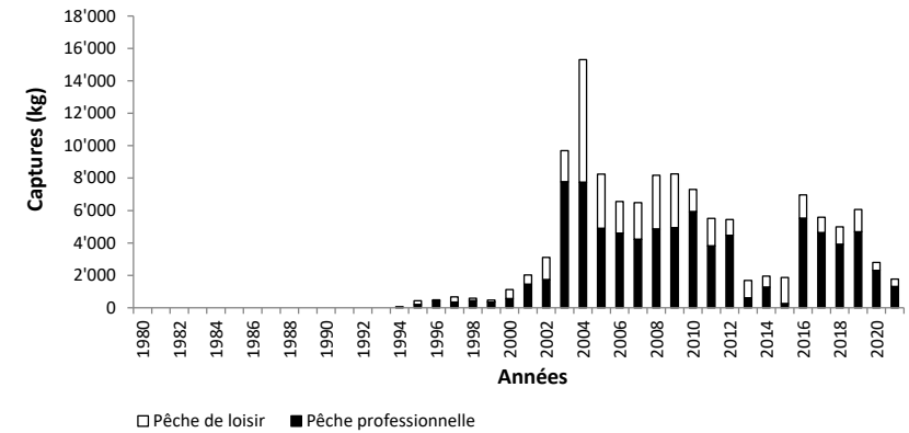
Historique des captures de sandres
