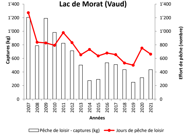
Captures et effort de pêche pour la pêche de loisir Lac de Morat (Vaud)
