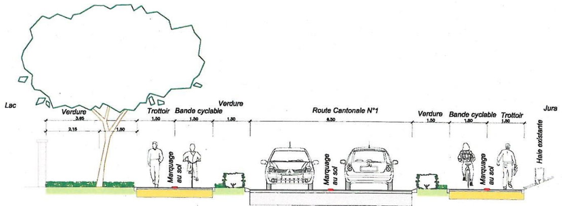
Profil chaussée avec deux zones mixtes :
