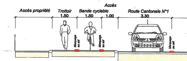
Profil d'accès à une propriété privée :
