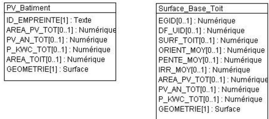
Figure 1. Diagramme de classes UML du Cadastre solaire
