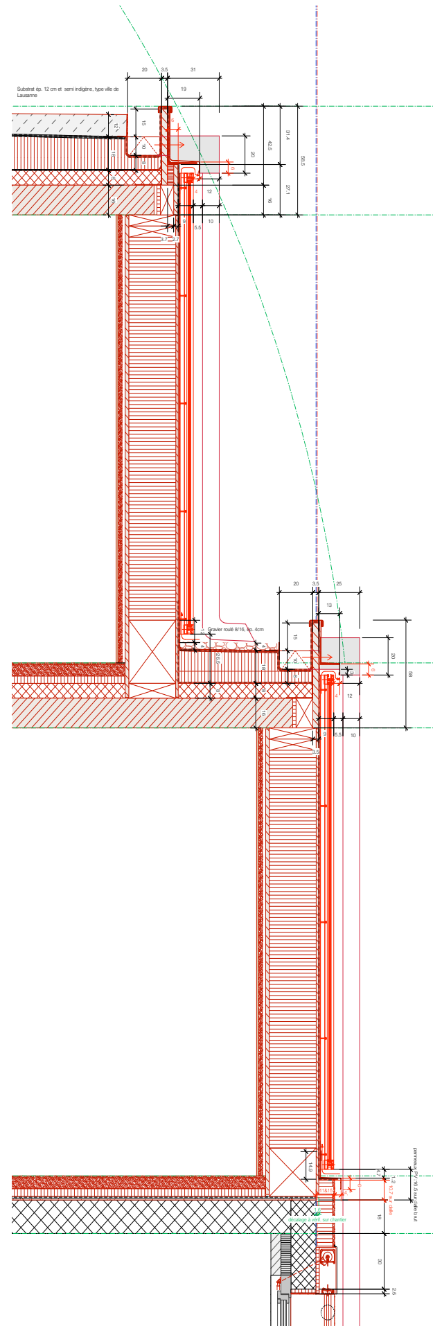
coupe-façade de détail
