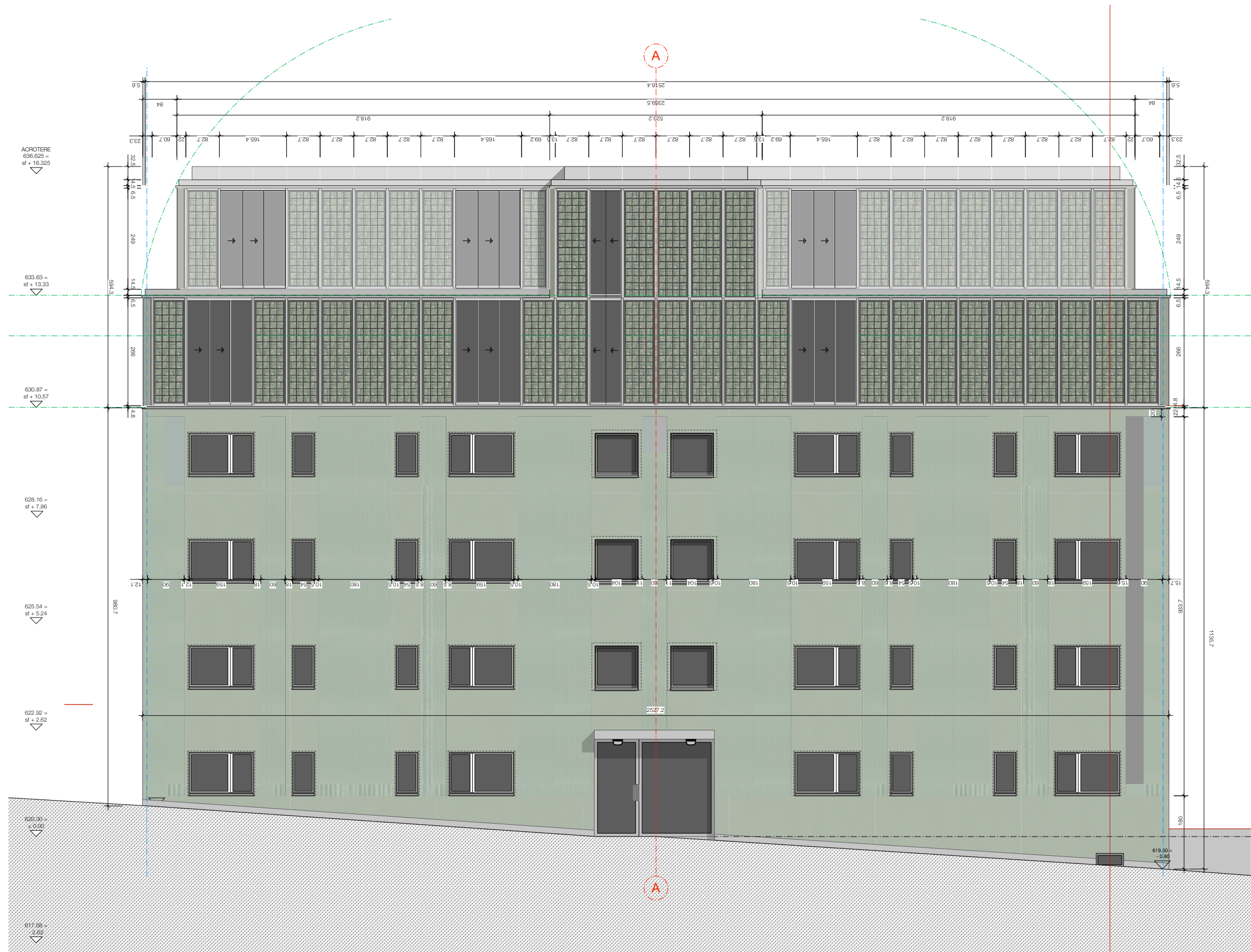
façade ouest
